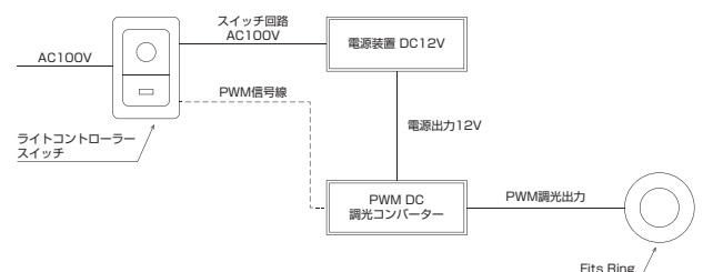
PWM 調光結線例
