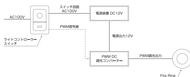
PWM 調光結線例
